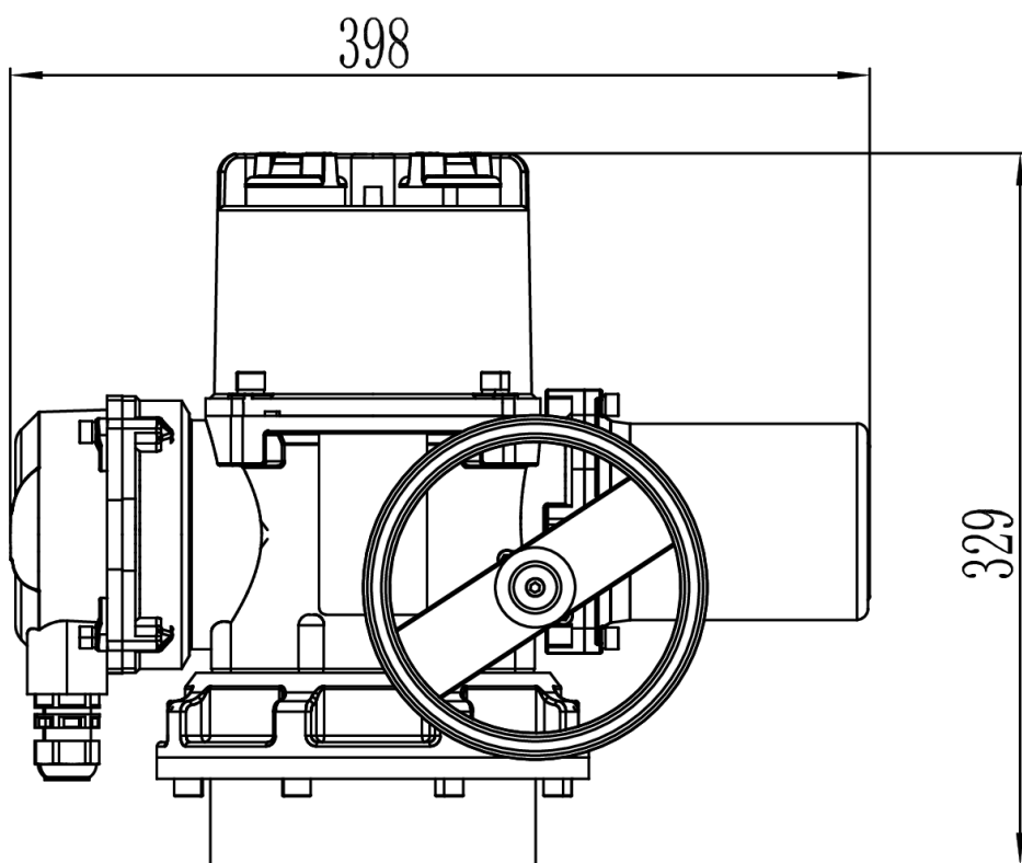
Габаритные размеры Электропривод DAUME FL 600-1800Nm
