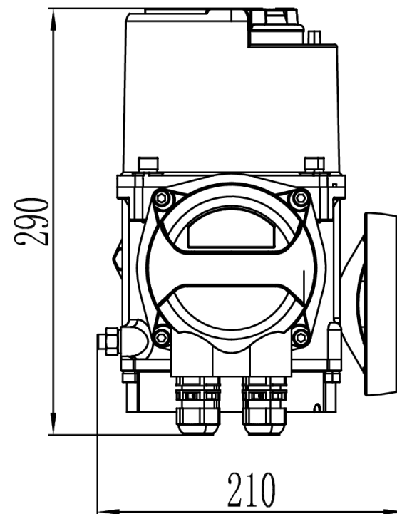
Габаритные размеры Электропривод DAUME FL 50-600Nm
