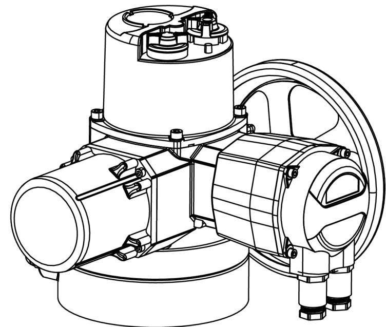
Габаритные размеры Электропривод DAUME FL 2500-5000Nm
