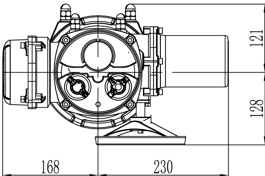
Габаритные размеры Электропривод DAUME FL 600-1800Nm
