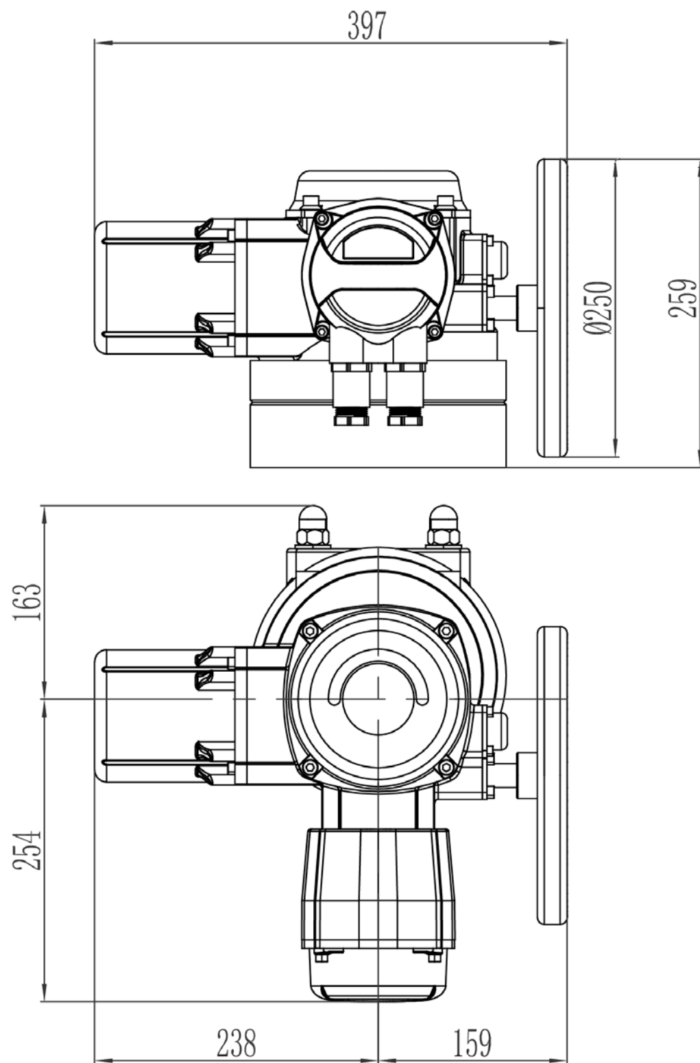
Габариты Электропривод DAUME F (Без блока) 2500-5000Nm
