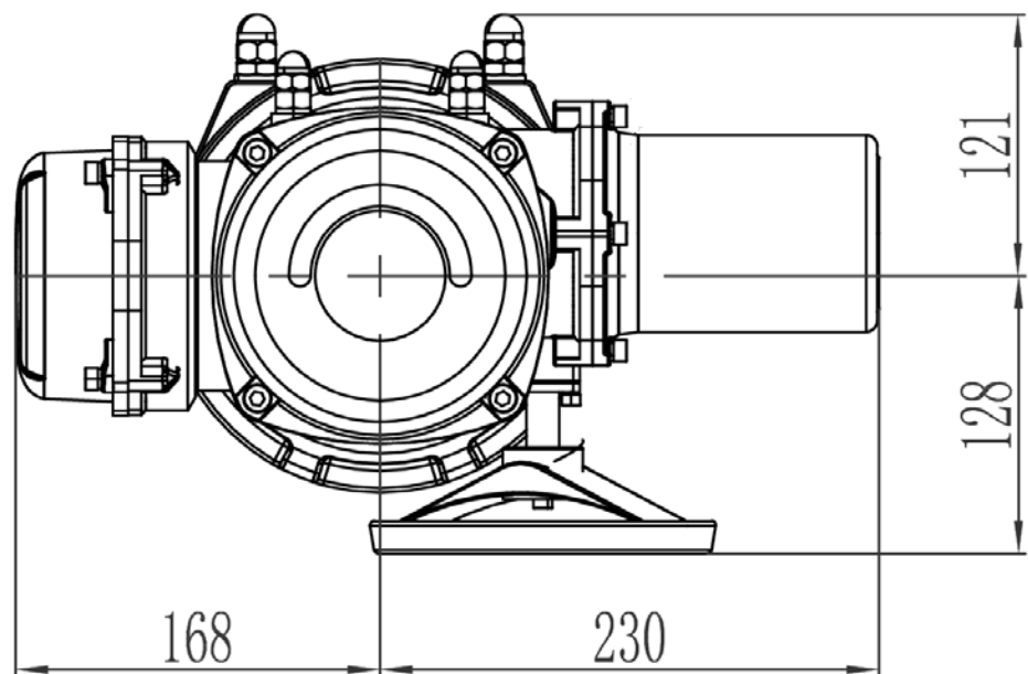
Габариты Электропривод DAUME F (Без блока) 600-1800Nm
